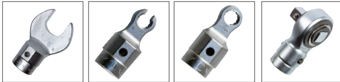
Ø16 mm Spigot Yuvarlak Girişli Uçlar / Ø16 mm Spigot End Fittings
